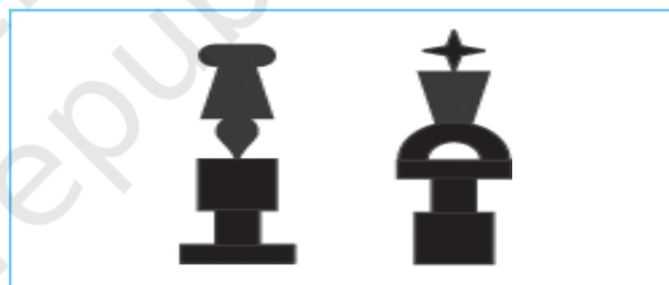
Fig.4.8 : Symmetry
